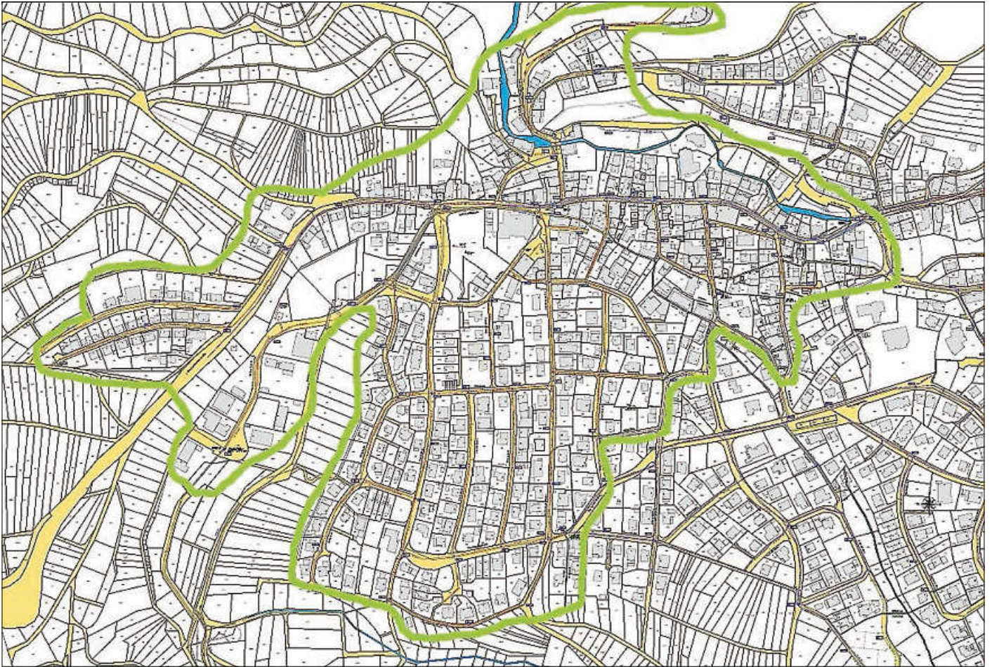
Wasserabstellung Tiefzone
