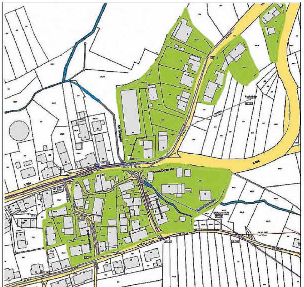
Wasserabstellung Mittelzone
